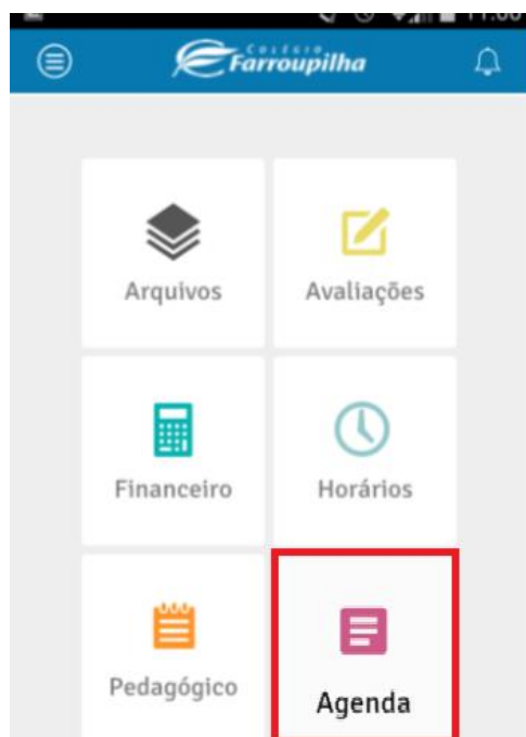
Figura 1 – Funcionalidade Agendas
